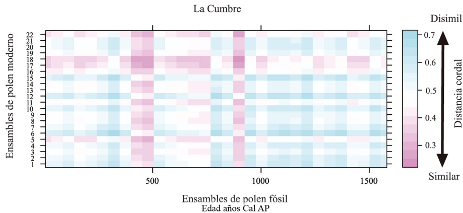
Figura 6. Índices de disimilitud de la distancia cordal en la secuencia de polen fósil y moderno a lo largo de ~ 1,580 años. La edad del sedimento en años calibrados antes del presente (años cal AP).
