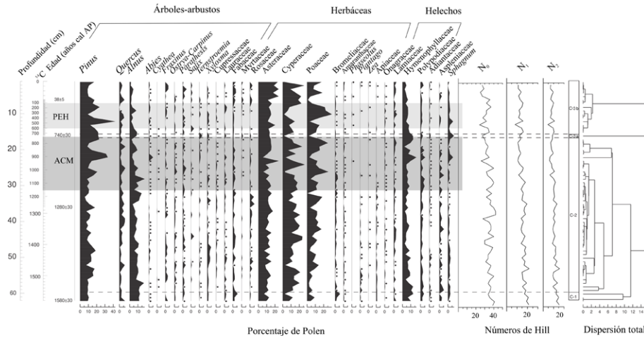
Figura 5. Diagrama de polen fósil del núcleo de sedimento CUM-N2 representando ~ 1,580 años de tasas de acumulación de especies del bosque de Pinus-Quercus-Abies . Se muestra la división de 3 zonas palinológicas mediante CONISS. La franja de color gris claro corresponde la Pequeña Edad de Hielo (PEH). La franja de color gris oscuro representa la Anomalia Climática Medieval (ACM). La escala muestra la profundidad en centímetros y la edad del sedimento en años calibrados antes del presente (años cal AP) (modificado de del Castillo-Batista et al., 2018).
