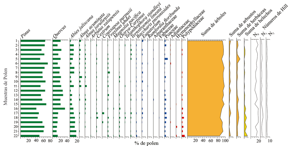
Figura 4. Diagrama de porcentajes de polen moderno del bosque de Pinus-Quercus-Abies en La Cumbre de Guadalupe.
