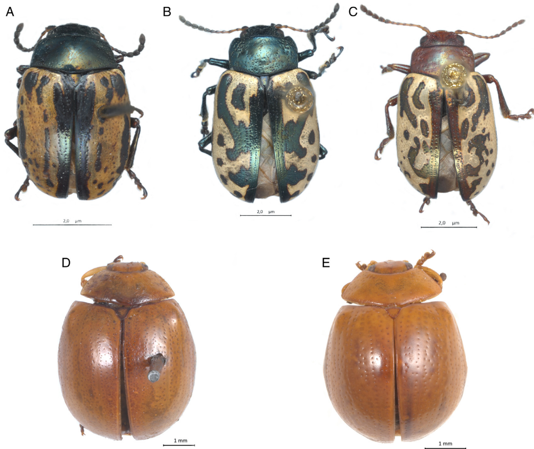
Figura 6. Vista dorsal de especies de Zygogramma , Pixis y Planagetes . A) Zygogramma obscurifasciata , B) Zygogramma signatipennis , C) Zygogramma piceicollis , D) Pixis indiga , E) Planagetes uniformis .
