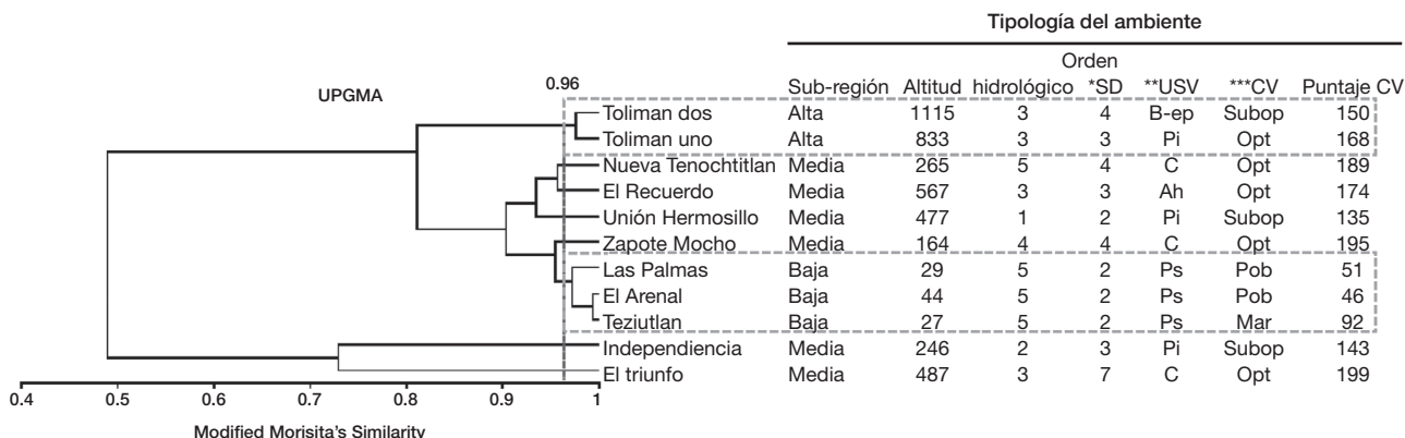
Figura 3. Índice de similitud de Morisita-Horn al 96% (línea discontinua) y tipología de ambiente (IMTA, 2013).
